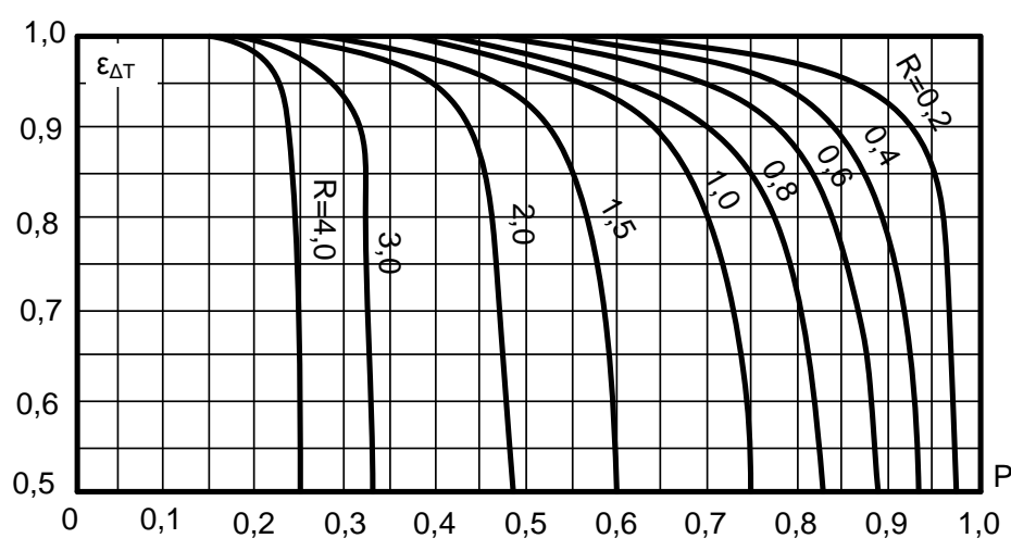
Рис. 5.3. \epsilon_{\Delta T} = f(P, R)
